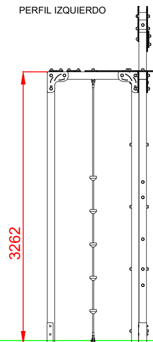
PERFIL IZQUIERDO
