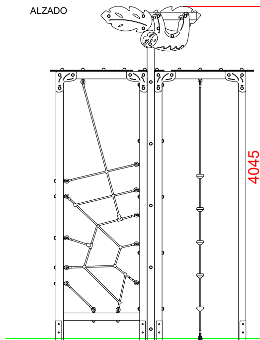
ALZADO
