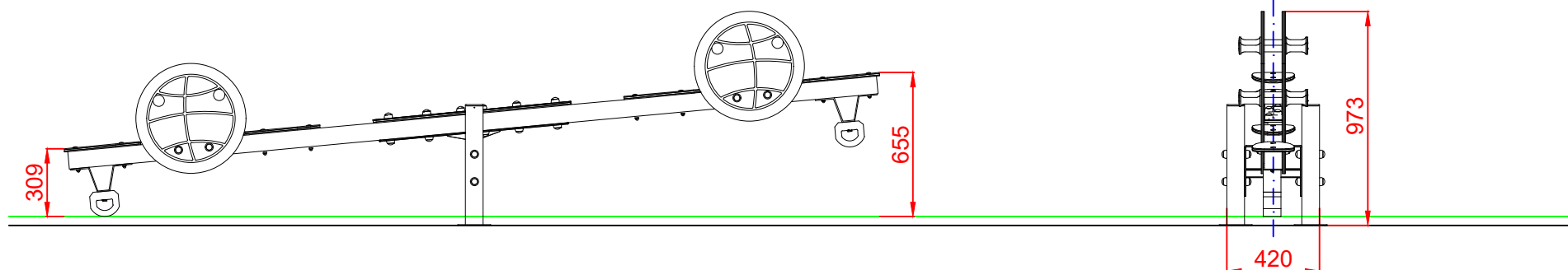
ALZADO
