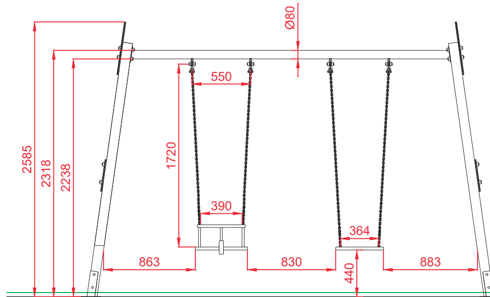
ALZADO
