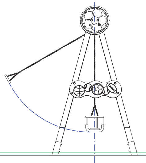
PERFIL IZQUIERDO
