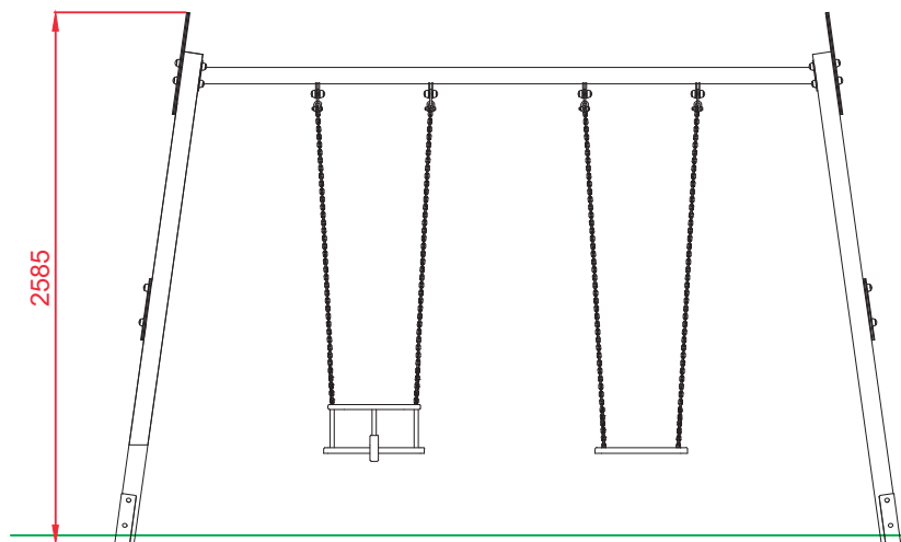
ALZADO
