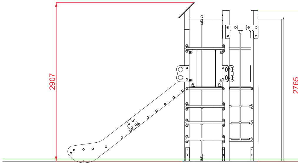
ALZADO
