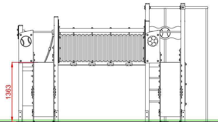
PERFIL IZQUIERDO
