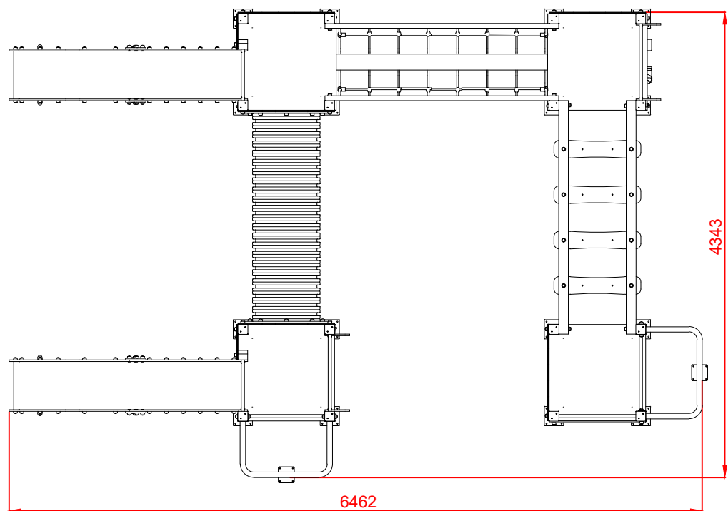
PLANTA
