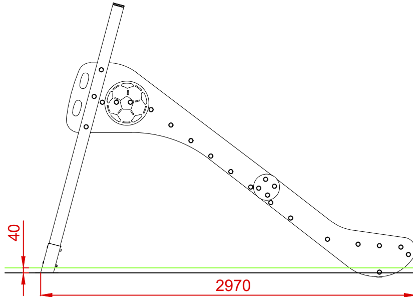
ALZADO
