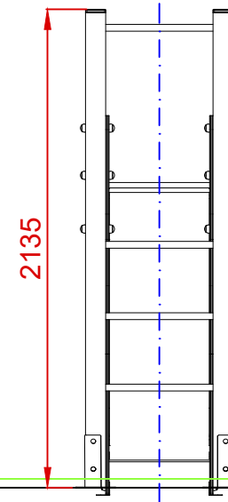
PERFIL IZQUIERDO
