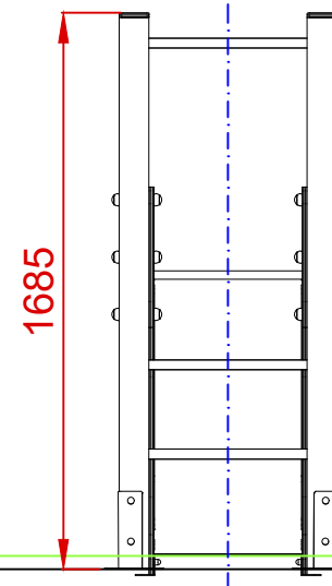
PERFIL IZQUIERDO
