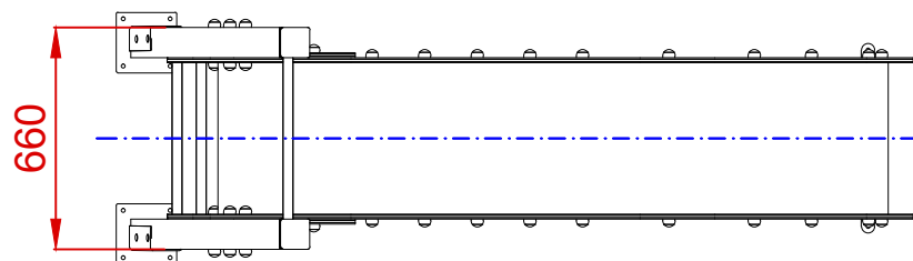
PLANTA
