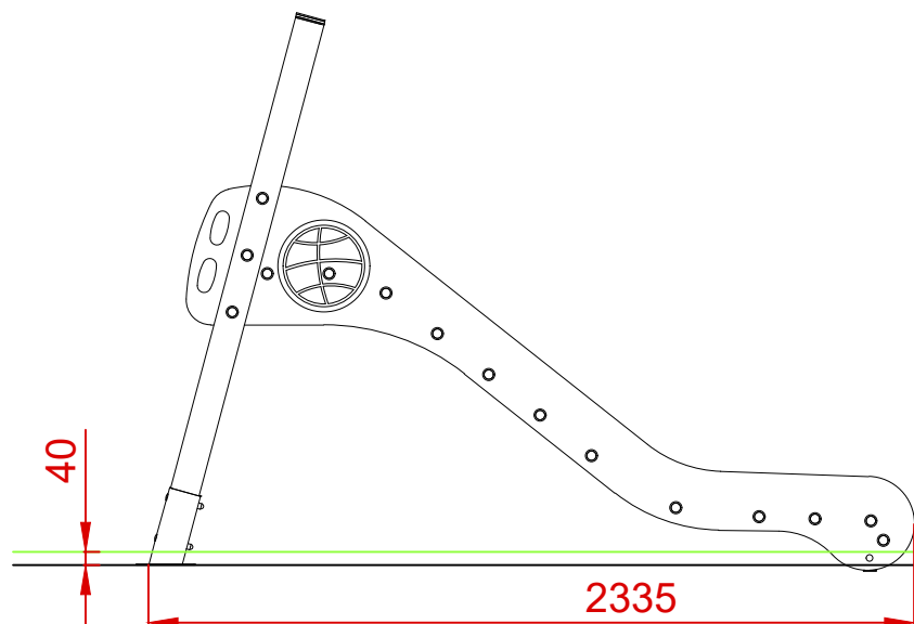
ALZADO
