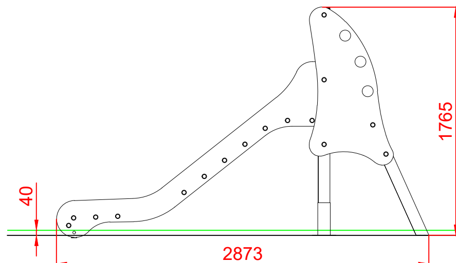
ALZADO
