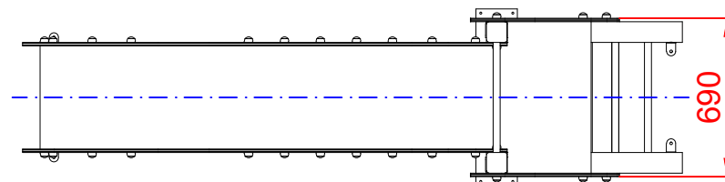
PLANTA
