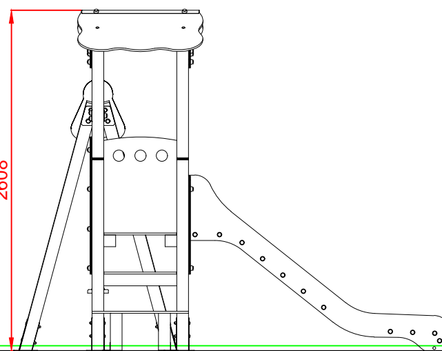
PERFIL IZQUIERDO
