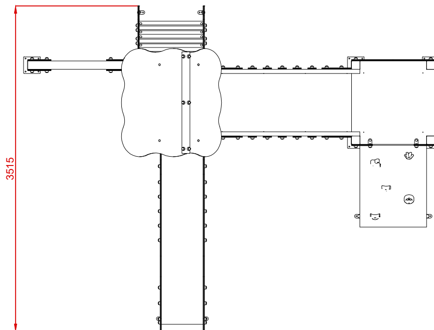
PLANTA
