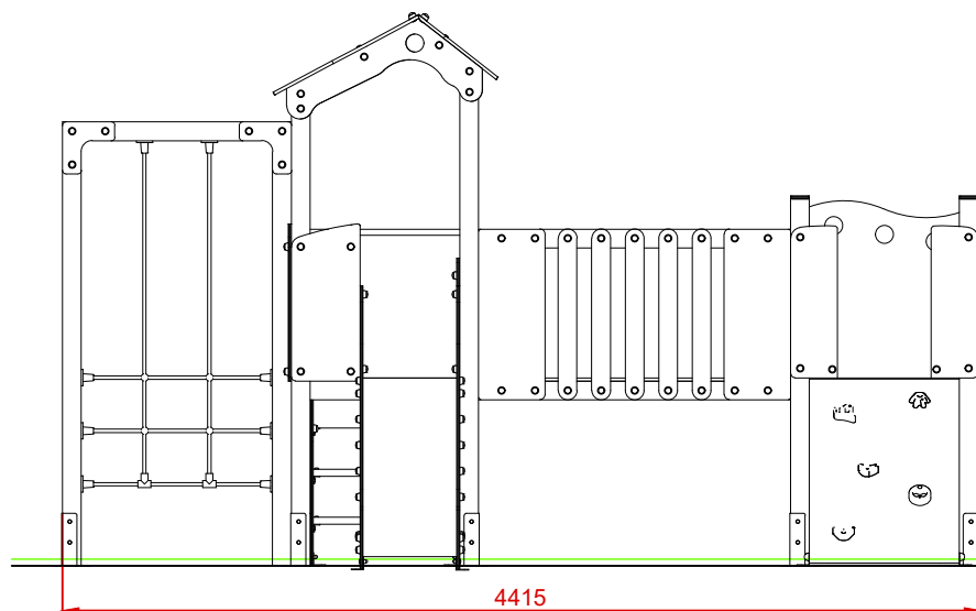
ALZADO
