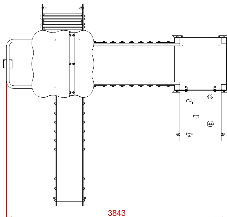
PLANTA
