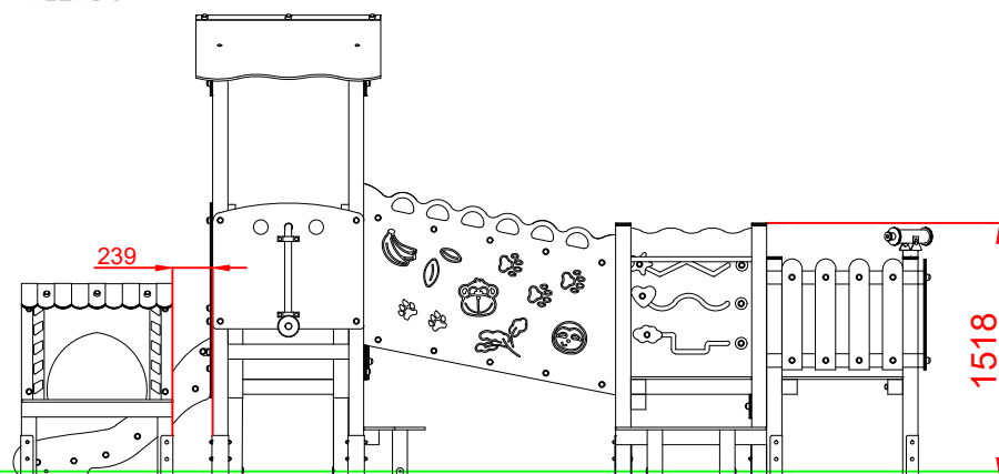
ALZADO
