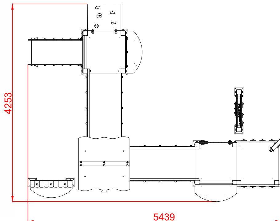
PLANTA
