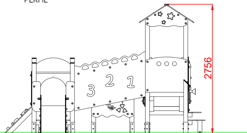
PERFIL
