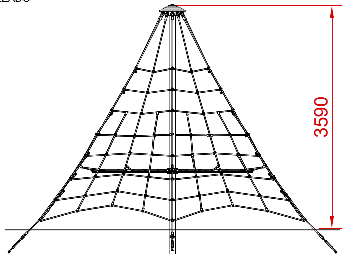
ALZADO
