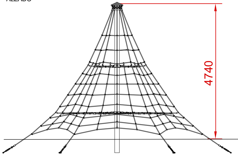
ALZADO
