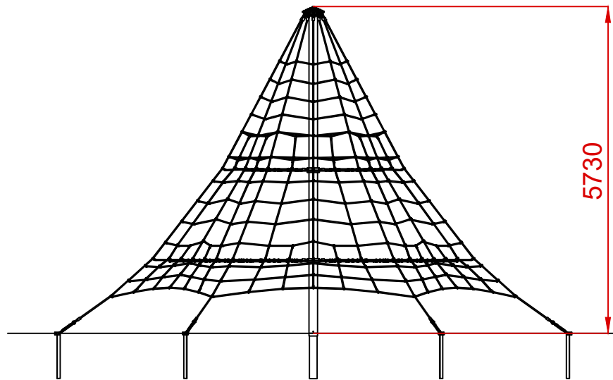
ALZADO
